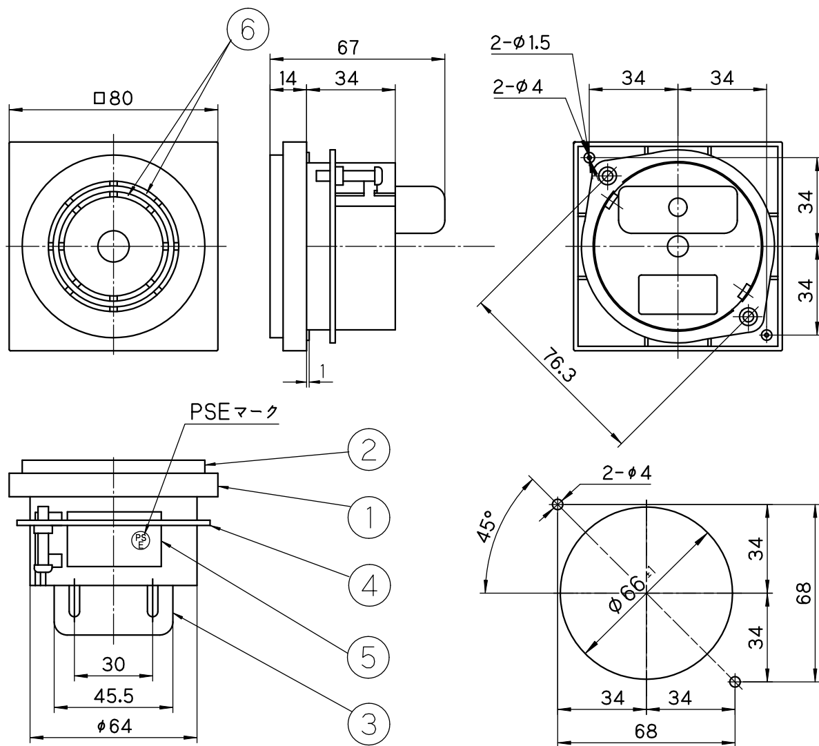
BZ-30 板金加工寸法
